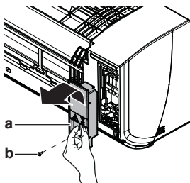
a Κάλυμμα συντήρησης b Βίδα καλύμματος συντήρησης
