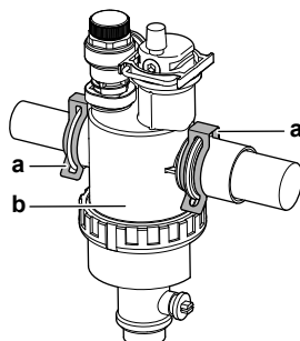
a Κλιπ b Μαγνητικό φίλτρο/διαχωριστή σωματιδίων
