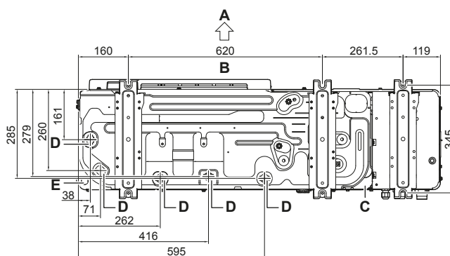
A Πλευρά εκκένωσης
