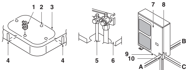
Εικόνα - Αγωγοί εξωτερικού χώρου σε τέσσερις κατευθύνσεις
