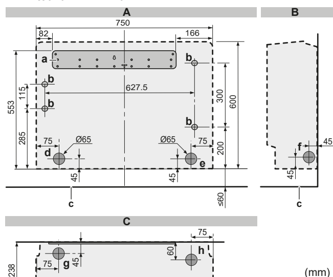
5-2 Σχέδιο εγκατάστασης εσωτερικής μονάδας: Επίτοιχη εγκατάσταση
