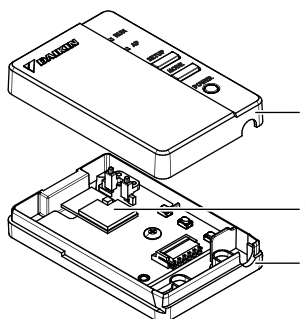
a Προστατευτικό περίβλημα b Σύνδεσμος c Κάτω περίβλημα
